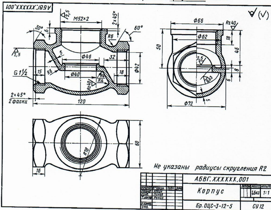
Лист 3 Рабочий чертёж корпуса вентиля
